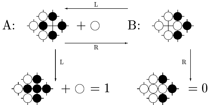
Figure 4: Ko.
